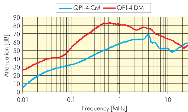
Рис. 6. Частотная характеристика подавления помех фильтра QPI-1 (верхняя кривая для дифференциальных помех, нижняя — для синфазных)
